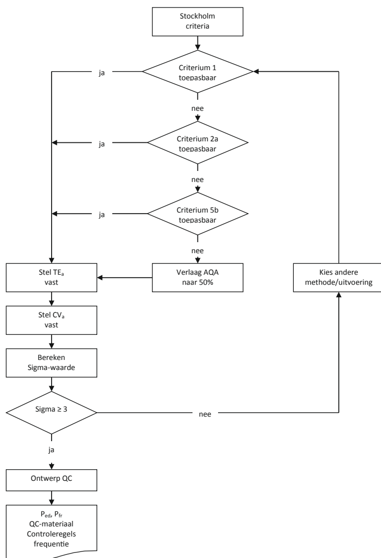
Figuur 6. Ontwerp IQC met behulp van Six Sigma.
