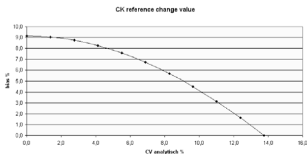
Figuur 7. De curve beschrijft combinaties van bias en CV_a , waarbij voldaan wordt aan de voorwaarde dat de grens van de RCV op P95,4% ligt (i.p.v. P97,5).
