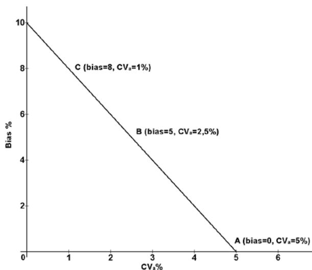
Figuur 3. Lineaire relatie tussen bias en analytische variatie. TE_a is vastgesteld op 10%, de z -waarde op 2 (dit zijn arbitrair gekozen waarden). Bij deze z -waarde valt 2,3% van de meetwaarden buiten de limiet van 10% maximale afwijking. Drie combinaties A, B en C voldoen aan de voorwaarden.
