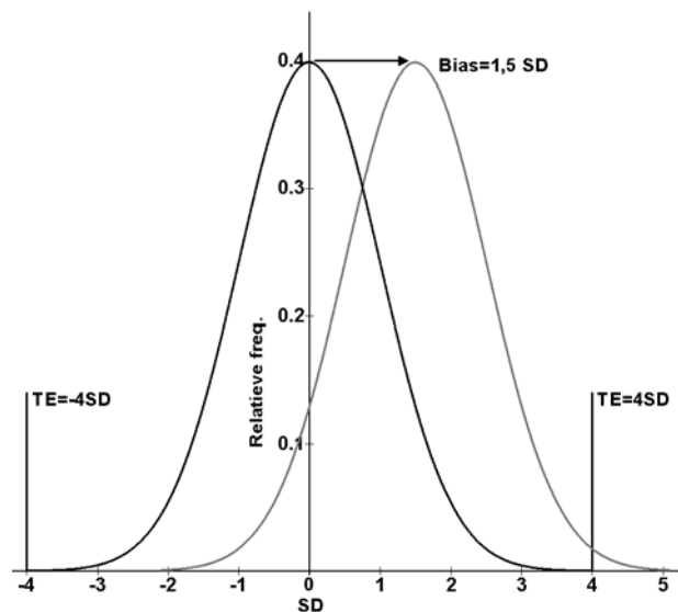
Figuur 1. Overschrijding van de \pm 4 \cdot SD limiet (4 Sigma proces) zonder bias: DPMO = 63; overschrijding met positieve bias van 1,5 SD: DPMO = 6.210.
