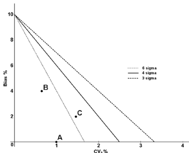
Figuur 5. Combinaties van bias en analytische variatie voor drie verschillende Sigma scores.
