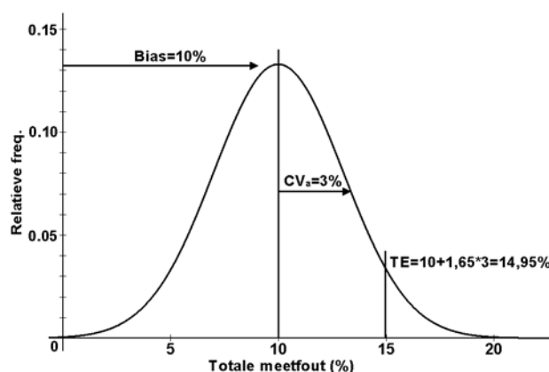
Figuur 2. Berekening van de totale meetfout op basis van bias en analytische variatie.
